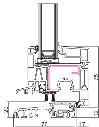
160x20 + SOGLIA ALU 548522
