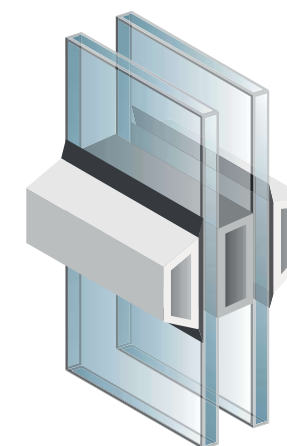
INGLESINE BIADESIVE CON IL DUPLEX
