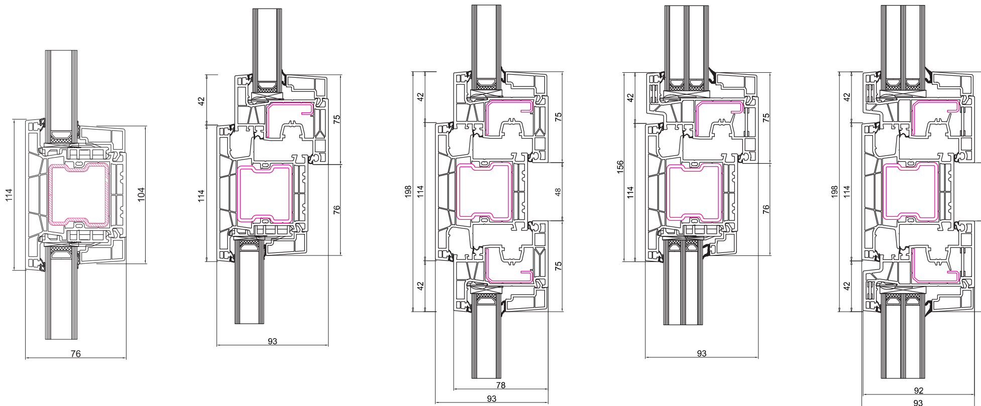
Fisso nel telaio 160x46
