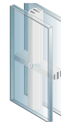
INGLESINE INCORPORATA CON PELLICOLA ANTIVIBRAZIONE
