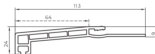
140219 (per finestra da restauro)
