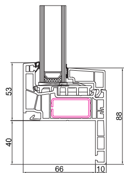
Fisso nel telaio 160x15
