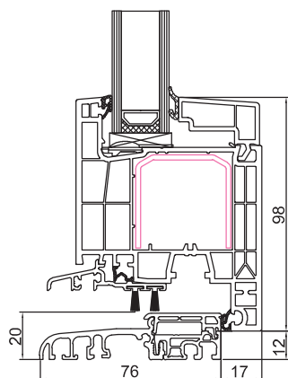
160x22 + SOGLIA ALU 548522
