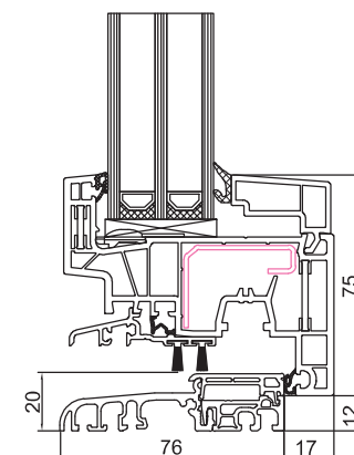
O60x27 + SOGLIA ALU 548522
