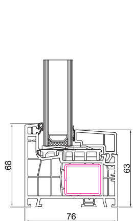
Fisso nel telaio 160x07
