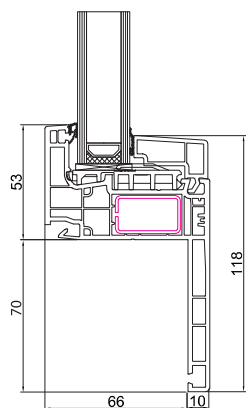
Fisso nel telaio 160x09
